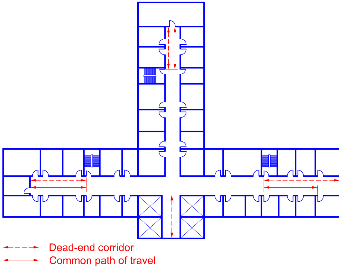
Diagram 2.5.1(b)-2
