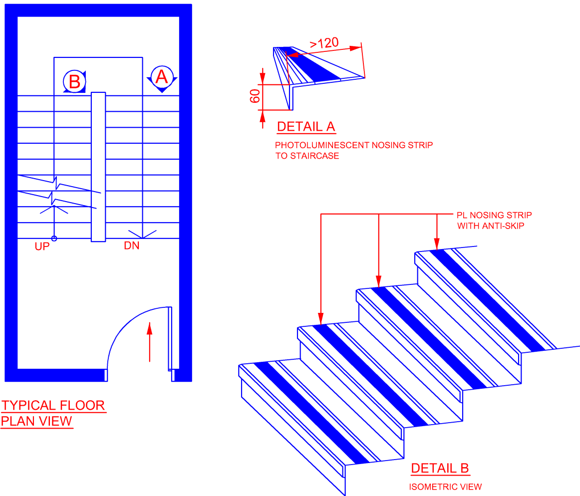
Diagram 2.10.4-1
