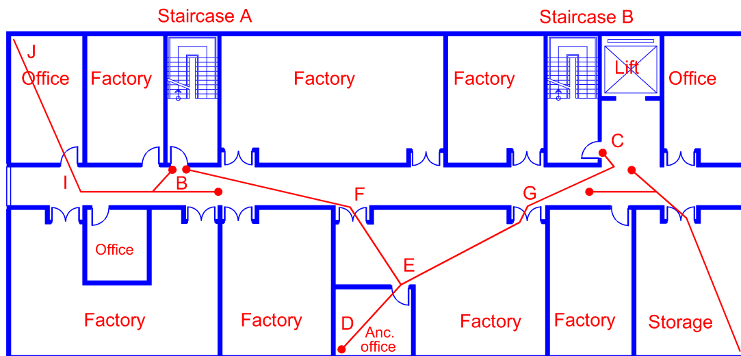
Diagram 2.2.12(b)-1
