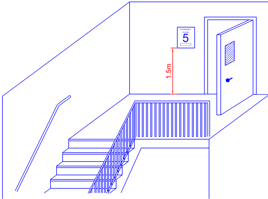
Diagram 2.3.1(b)-3
