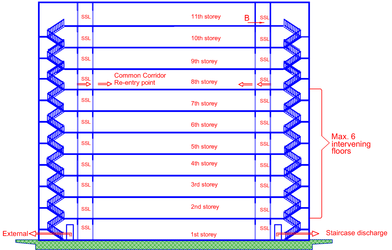
Diagram 2.3.9(l)-3
