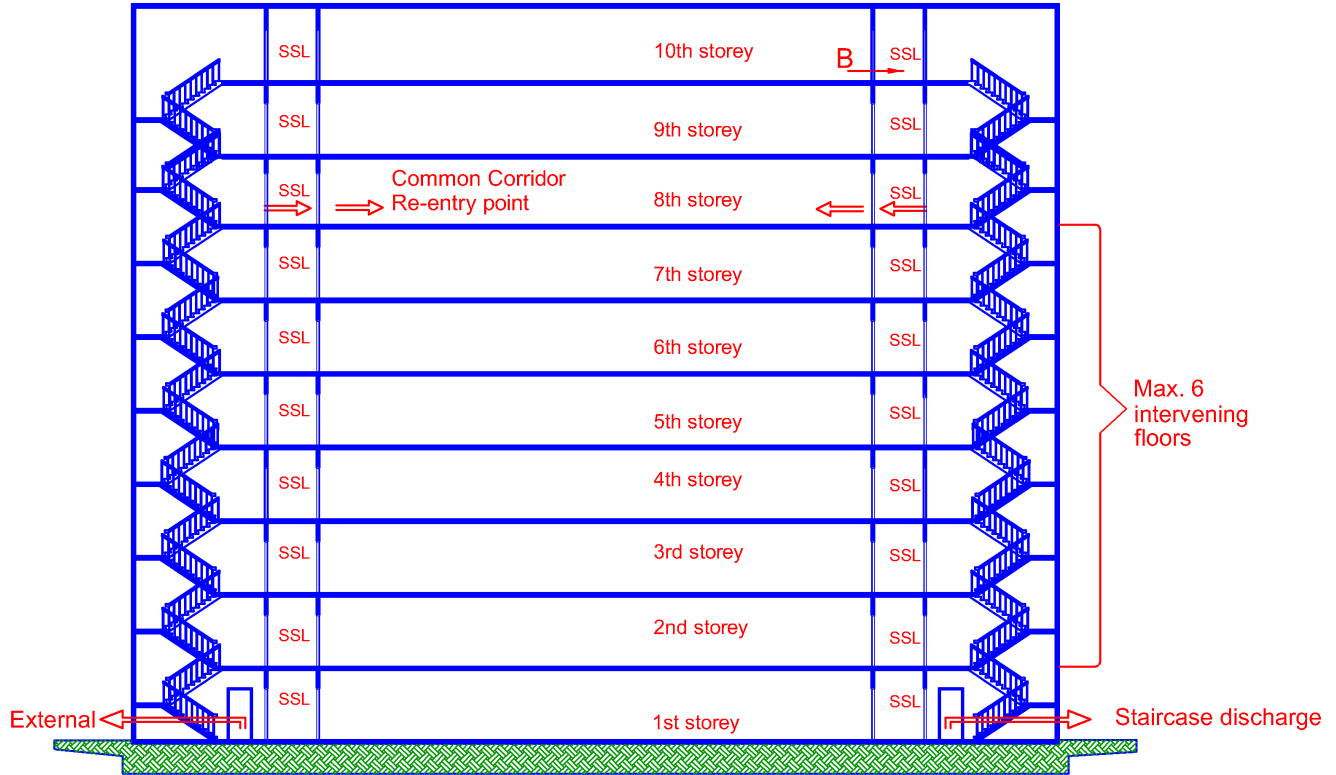
Diagram 2.3.9(l)-2
