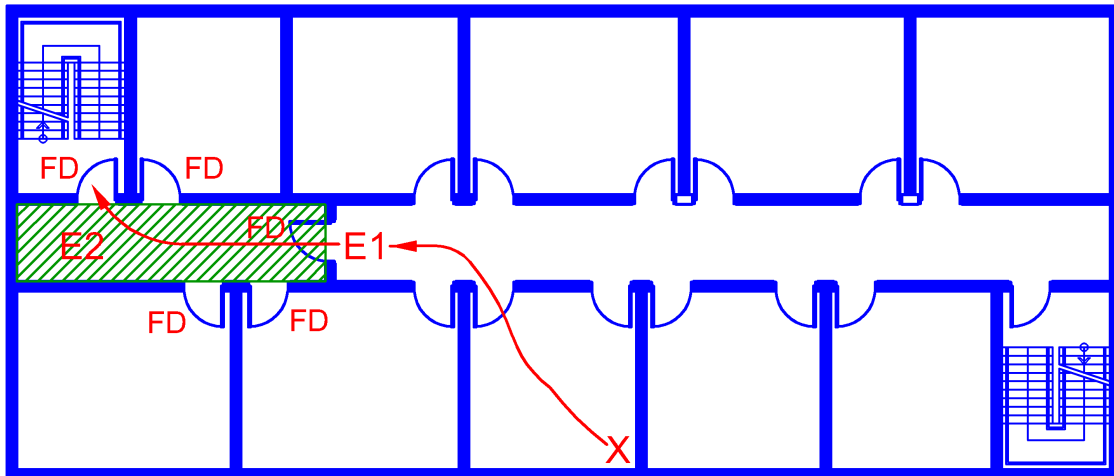
Diagram 2.3.2(b)-2
