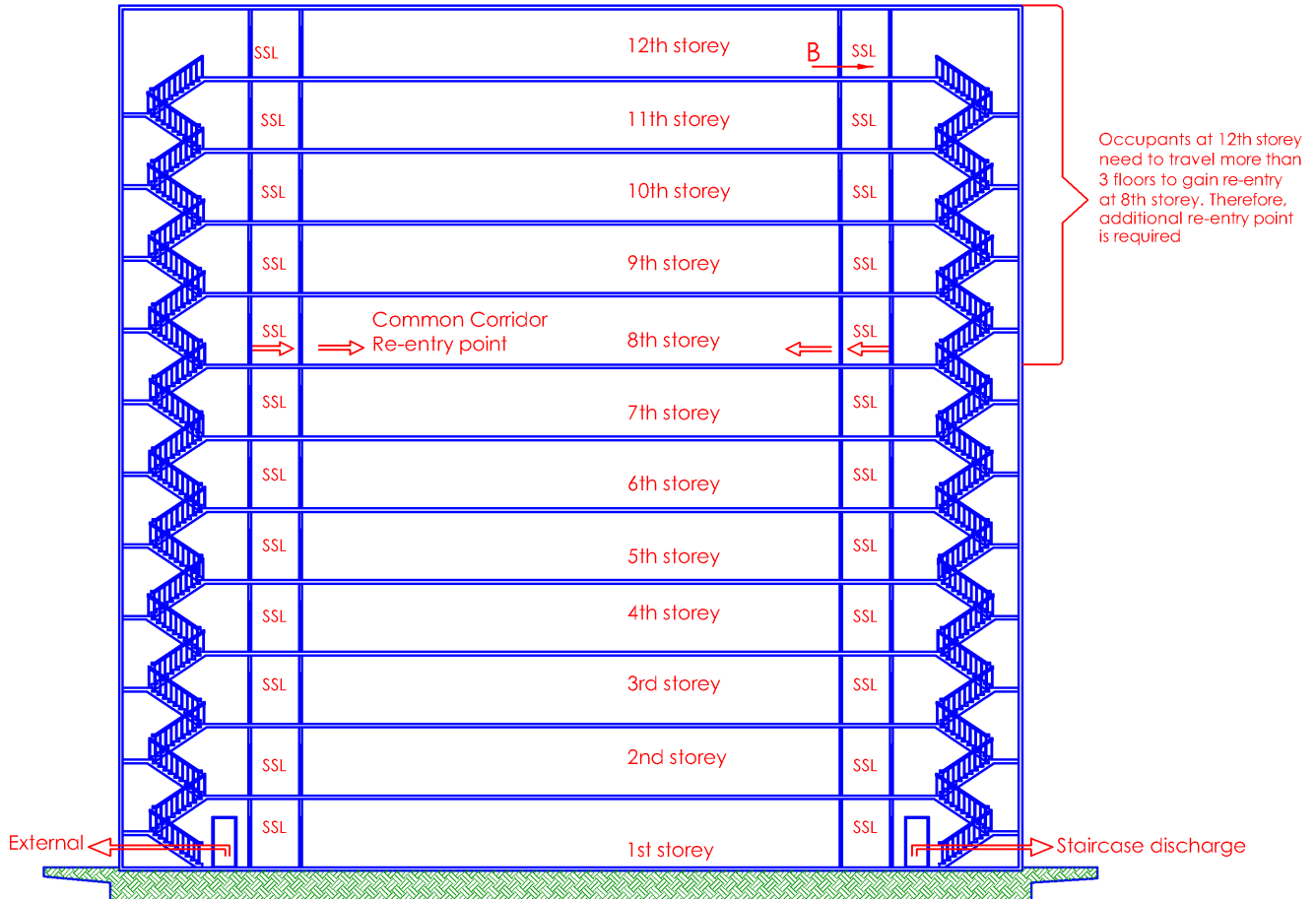
Diagram 2.3.9(l)-4
