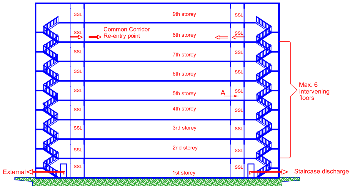
Diagram 2.3.9(l)-1
