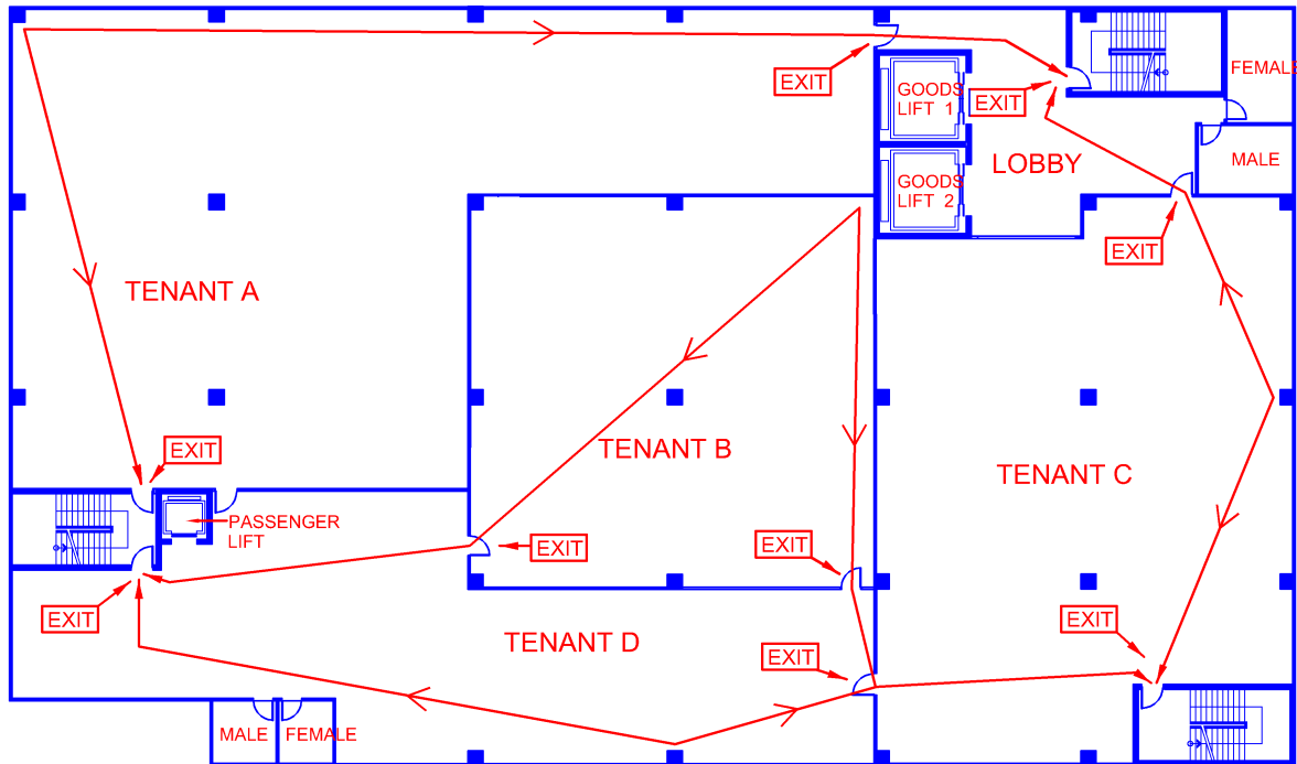
Diagram 2.2.12(b)-3
