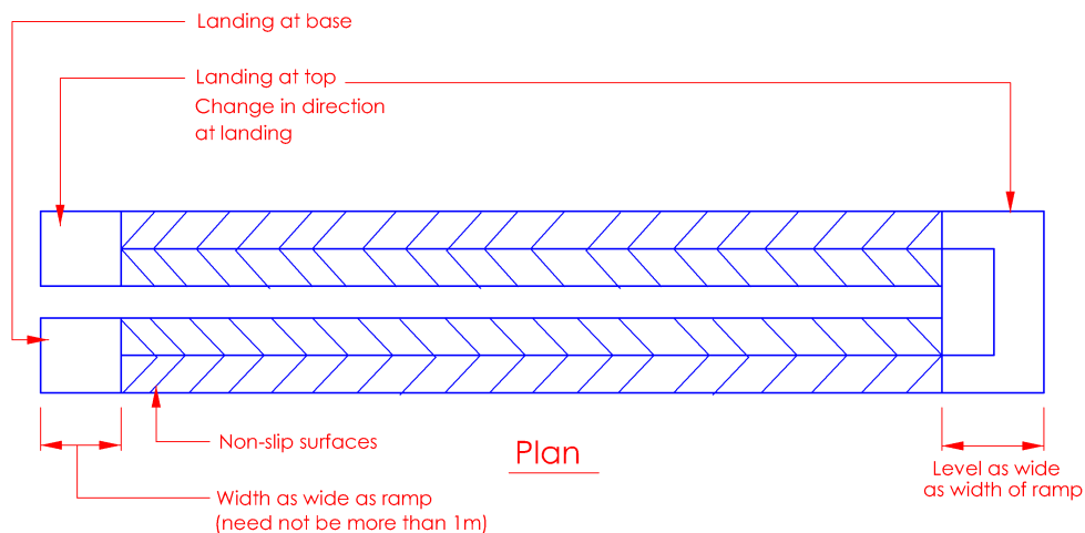
Diagram 2.3.8(c)
