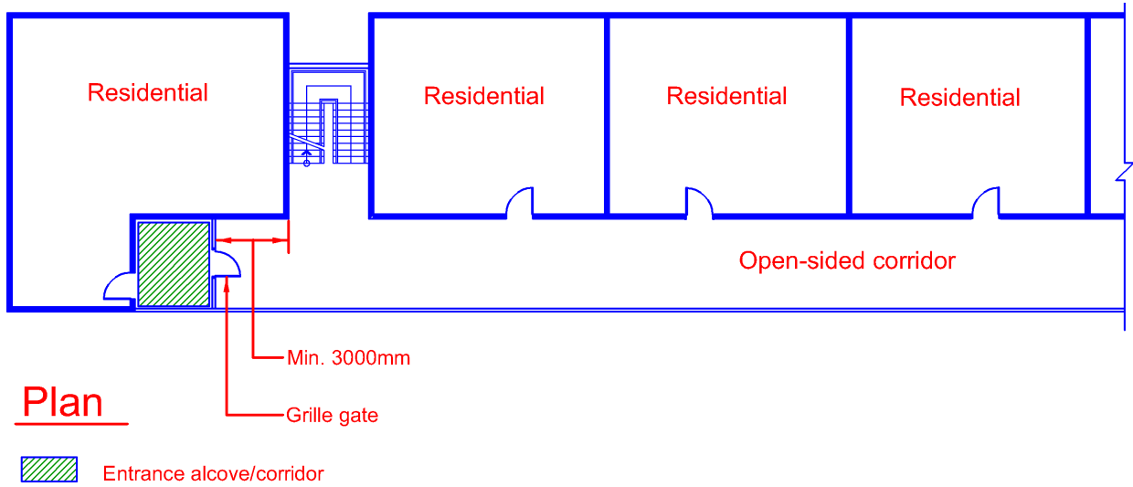
Diagram 2.3.9(g)-3
