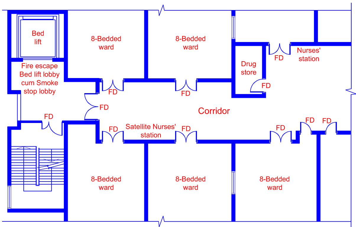
Diagram 2.5.1 (a)(viii)
