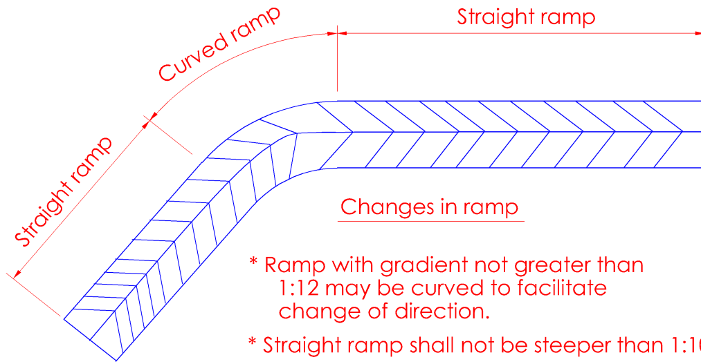
Diagram 2.3.8(b)-1
