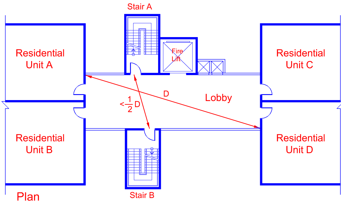
Diagram 2.2.12(c)-3
