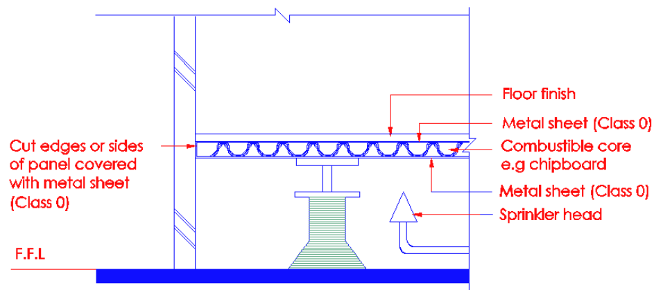
Diagram 3.11.8(e)
