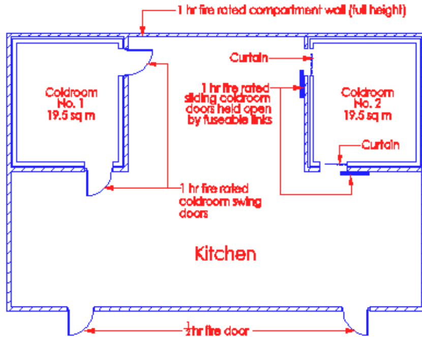
Diagram 3.2.5(m)-3
