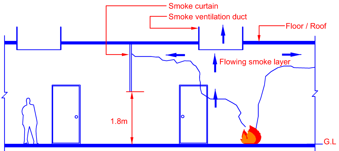
Elevation A
