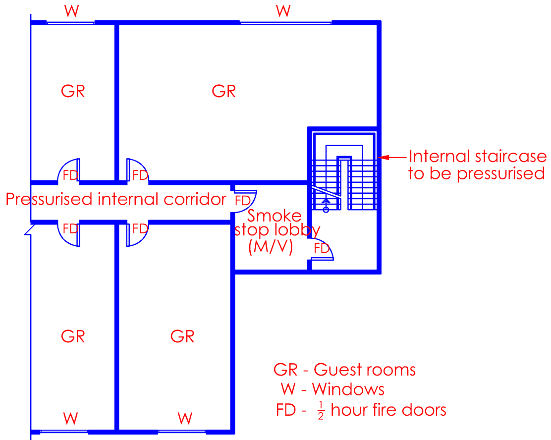
Diagram 7.3.1-2
