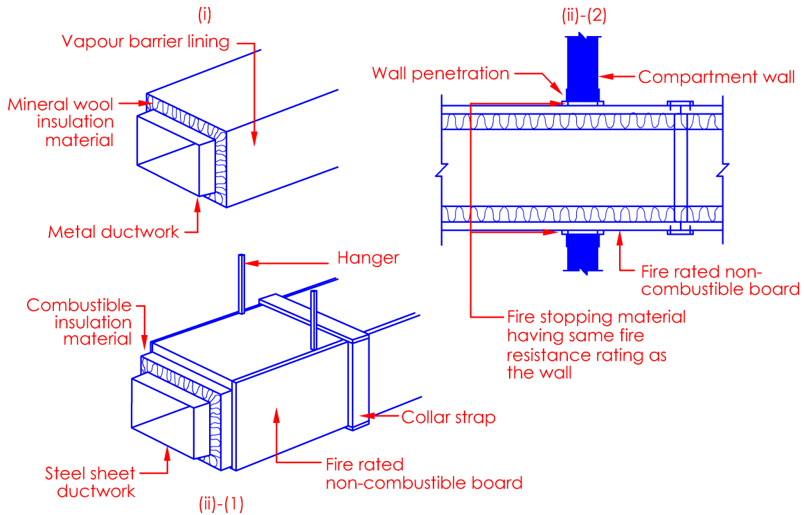
Diagram 7.1.1(b)
