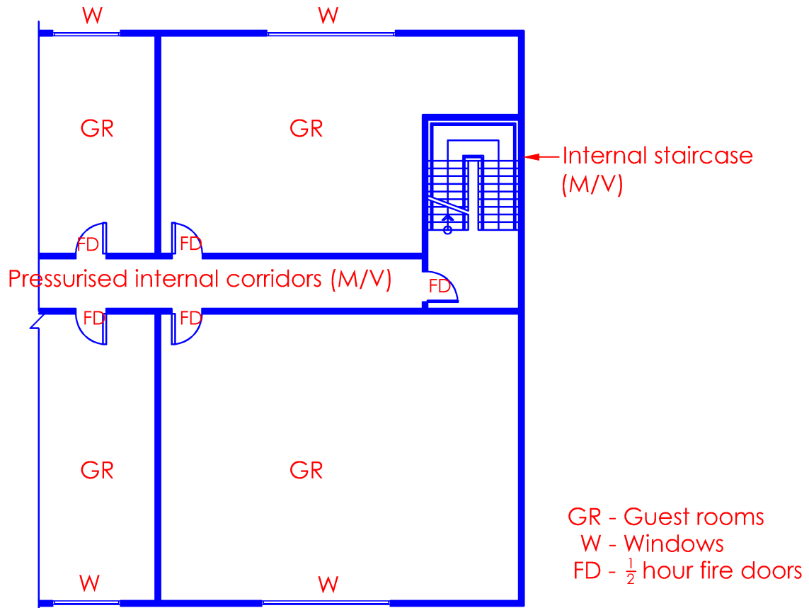
Diagram 7.3.1-6
