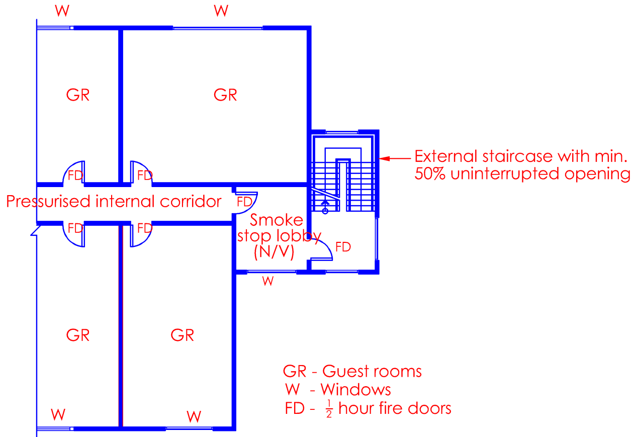
Diagram 7.3.1-4
