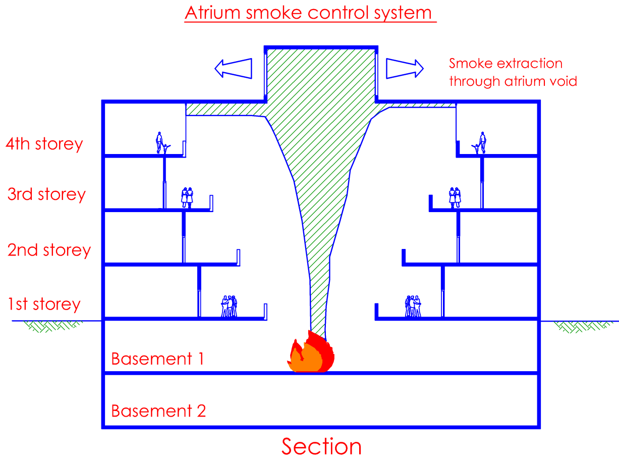
Diagram 7.5.1
