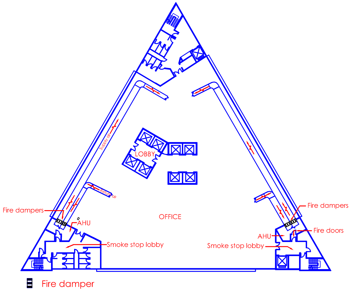
Diagram 7.1.1(e)-3
