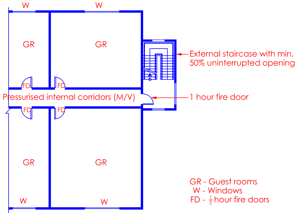
Diagram 7.3.1-5
